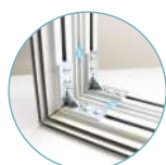
Montagem de secções, ângulo reto com conectores de aparafusar
